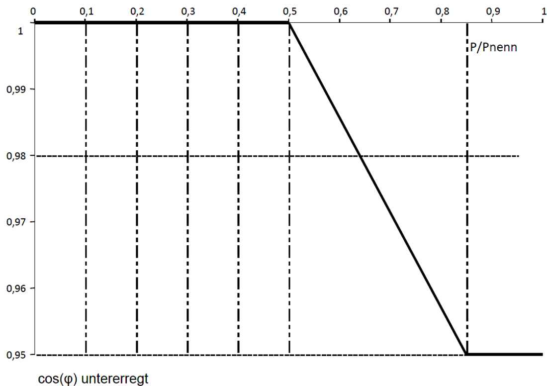
Abbildung 1: \cos(\varphi) = f(P) -Kennlinie für Erzeugungsanlagen am Mittelspannungsnetz
